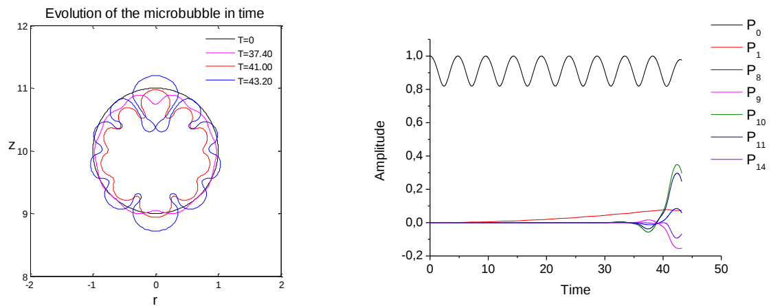
Διάγραμμα 4- 3: Χρονική εξέλιξη του σχήματος της φυσαλίδας (αριστερά), διάγραμμα χρονικής εξέλιξης των ιδιομορφών σχήματος της φυσαλίδας (δεξιά) για \varepsilon=0.5 και d=5 .
