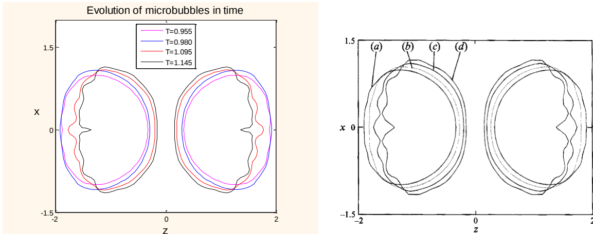
Διάγραμμα 3- 1: Χρονική εξέλιξη σχήματος των δύο φυσαλίδων στο τελικό στάδιο της προσομοίωσης, για d^* = 4 \text{ mm} . Αποτέλεσμα προσομοίωσης (αριστερά), αντίστοιχο γράφημα από τη βιβλιογραφία (δεξιά).
