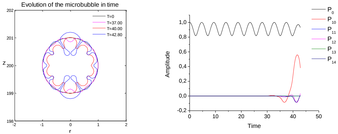
Διάγραμμα 4- 2: Χρονική εξέλιξη του σχήματος της φυσαλίδας (αριστερά), διάγραμμα χρονικής εξέλιξης των ιδιομορφών σχήματος της φυσαλίδας (δεξιά) για \varepsilon=0.5 και d=100 .
