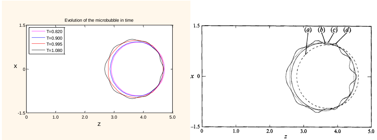
Διάγραμμα 3- 3: Χρονική εξέλιξη σχήματος των δύο φυσαλίδων στο τελικό στάδιο της προσομοίωσης, για d^*=8\text{mm} . Αποτέλεσμα προσομοίωσης (αριστερά), αντίστοιχο γράφημα από τη βιβλιογραφία (δεξιά).
