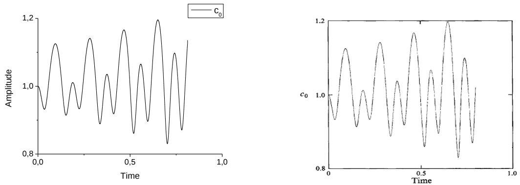
Διάγραμμα 3- 8: Διαγράμματα ταλαντώσεων όγκου της φυσαλίδας, για d^*=8\text{mm} και \nu_f^*=1503 \text{ Hz} . Αποτελέσματα της προσομοίωσης (αριστερά), αντίστοιχα διαγράμματα από τη βιβλιογραφία (δεξιά).
