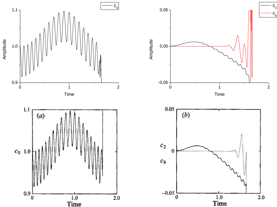
Διάγραμμα 3- 6: Χρονική μεταβολή των συντελεστών Legendre c_0 , c_2 και c_9 , για d^*=8\text{mm} και \nu_f^*=152\text{ Hz} . Αποτελέσματα της προσομοίωσης (πάνω), αντίστοιχα αποτελέσματα από τη βιβλιογραφία (κάτω).
