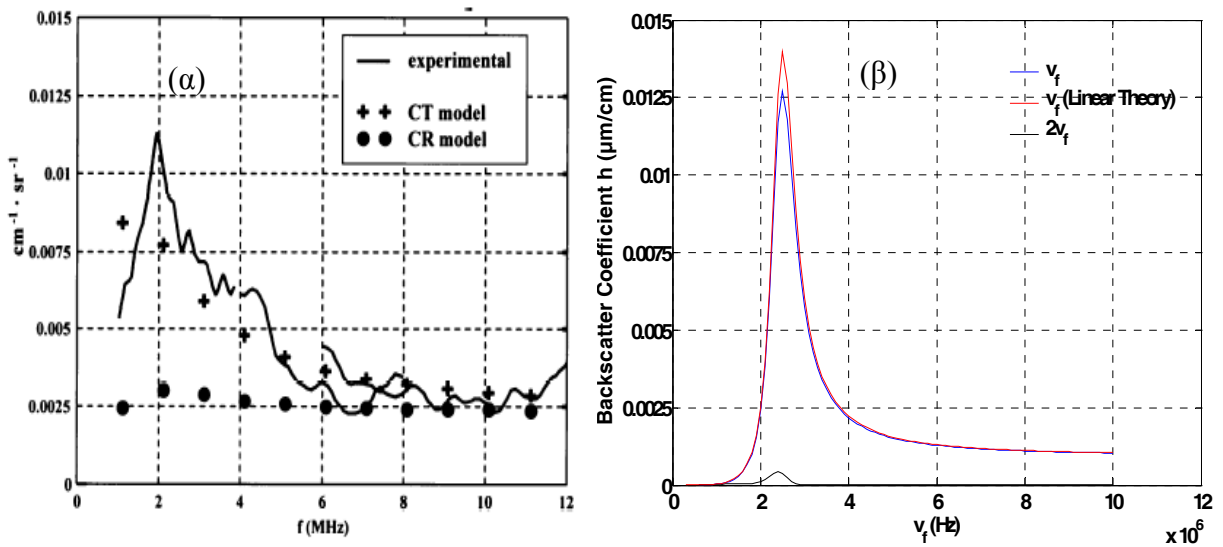
Σχήμα 13. Ο συντελεστής h (backscatter coefficient) σα συνάρτηση της εξωτερικής συχνότητας α) Πείραμα των Jean – Marie Gorce et al, β) Παρόν αριθμητικό μοντέλο. Δεδομένα προσομοίωσης: \gamma=1.4 , P_{\text{inf}}=101325 \text{ Pa} , \rho_l=998 \text{ kg/m}^3 , s_1=0.04 \text{ kg/s}^2 , s_2=0.005 \text{ kg/s}^2 , G_s=36.67 \text{ MPa} , \mu_s=0.5968 \text{ kgm}^{-1}\text{s}^{-1} , \delta=15 \cdot 10^{-9} \text{ m} , E_{\text{inf}}=0.5 . u_r(t=0)|_{r=1} = u_r(t=0)|_{r=a_{\text{bol}}} = 0
