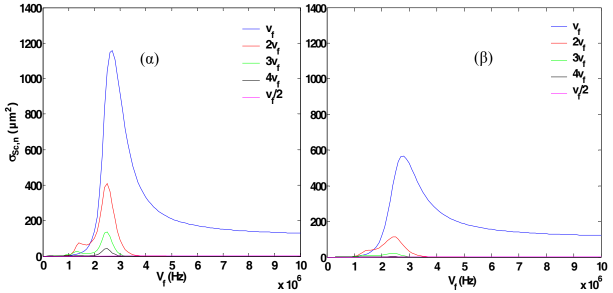
Σχήμα 8. Το \sigma_{Sc,n} σε συνάρτηση της εξωτερικής συχνότητας για α) νερό ( C_I=1500 m/s, \mu_I=0.001 kgm -1 s -1 ) β) αίμα ( C_I=500 m/s, \mu_I=0.004 kgm -1 s -1 ). Δεδομένα προσομοίωσης: \gamma=1.4 , P_{inf}=101325 Pa, \rho_I=998 kg/m 3 , s_1=0.04 kg/s 2 , s_2=0.005 kg/s 2 , \alpha=3*10^{-6} m, G_s=35 MPa, \mu_s=0.6 kgm -1 s -1 , \delta=15*10^{-9} m, E_{inf}=2.05 . u_r(t=0)|_{r=1} = u_r(t=0)|_{r=a_{bal}} = 0
