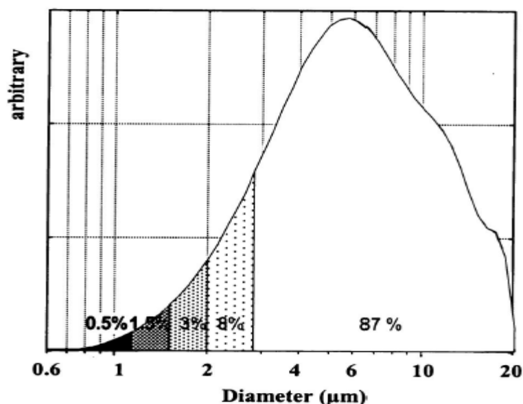
Σχήμα 12. Η συγκέντρωση κ.ο. των μικροφουσαλίδων στο πείραμα των Jean – Marie Gorce et al.
