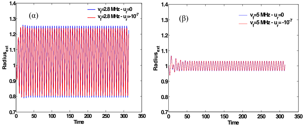
Σχήμα 9. Η εξωτερική ακτίνα της μικροφουσαλίδας σε συνάρτηση του χρόνου με και χωρίς παραμένουσες τάσεις στη μεμβράνη α) σε συντονισμό β) εκτός συντονισμού. Δεδομένα προσομοίωσης: \gamma=1.4 , P_{inf}=101325 Pa, \rho_l=998 kg/m 3 , s_1=0.04 kg/s 2 , s_2=0.005 kg/s 2 , \mu_l=0.001 kgm -1 s -1 , C_l=1500 m/s, \mu_s=0.6 kgm -1 s -1 , G_s=35 MPa, \alpha=3*10^{-6} m, \delta=15*10^{-9} m, E_{inf}=0.05 .
