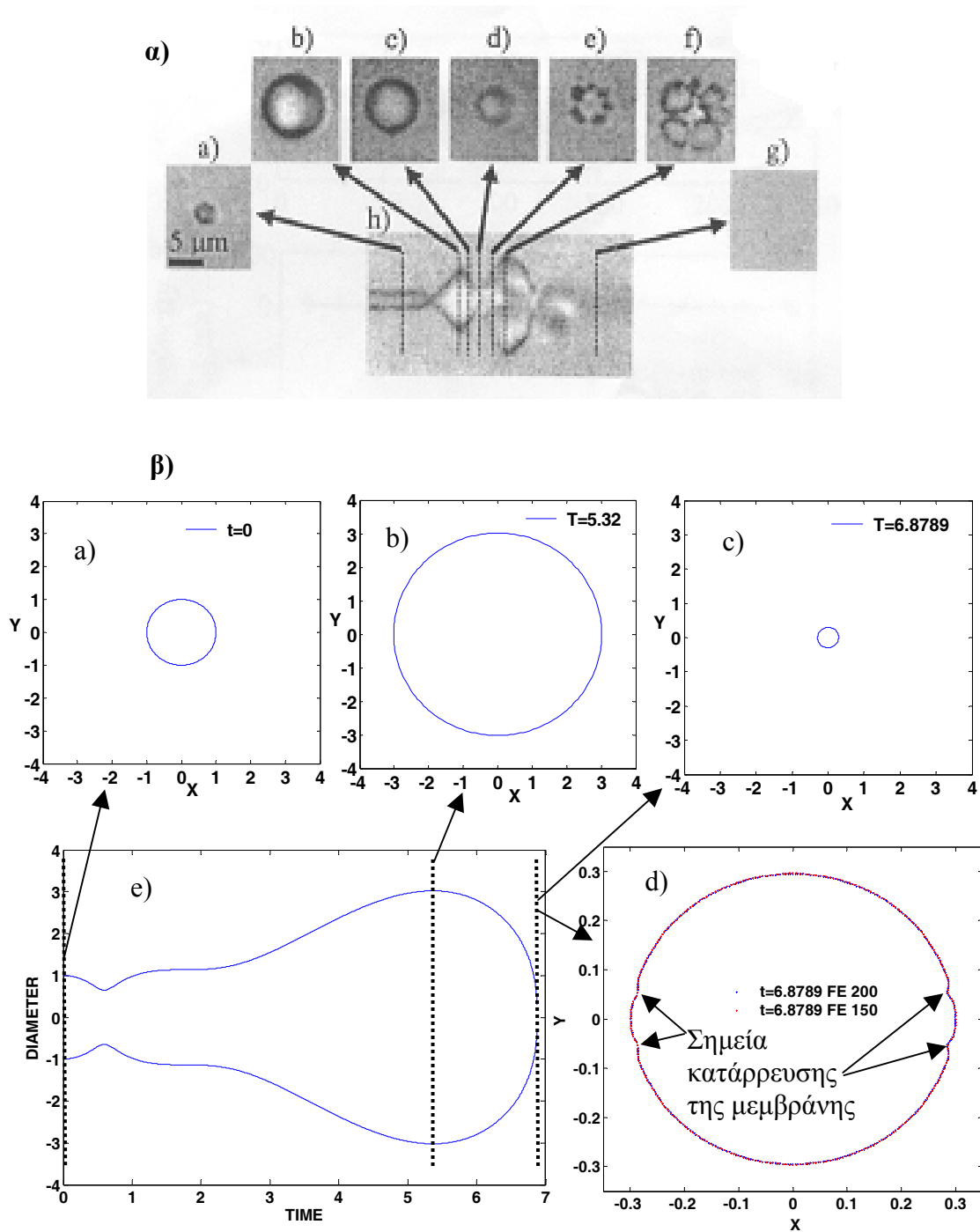
Σχήμα 5. Η δυναμική συμπεριφορά της μικροφυσαλίδας και ο τρόπος κατάρρευσης της α) πειραματικά αποτελέσματα από τους James E.Chomas et al. β) αριθμητική προσομοίωση. Δεδομένα προσομοίωσης: R_{bal}=1.5 \mu m , G_s=18 \text{ MPa} , \alpha=0.5 , \delta=15 \text{ nm} , \rho_l=998 \text{ kg/m}^3 , P_{st}=1 \text{ atm} , \nu_f=2.4 \text{ MHz} , \epsilon_{int}=12 , \gamma=1.4 .
