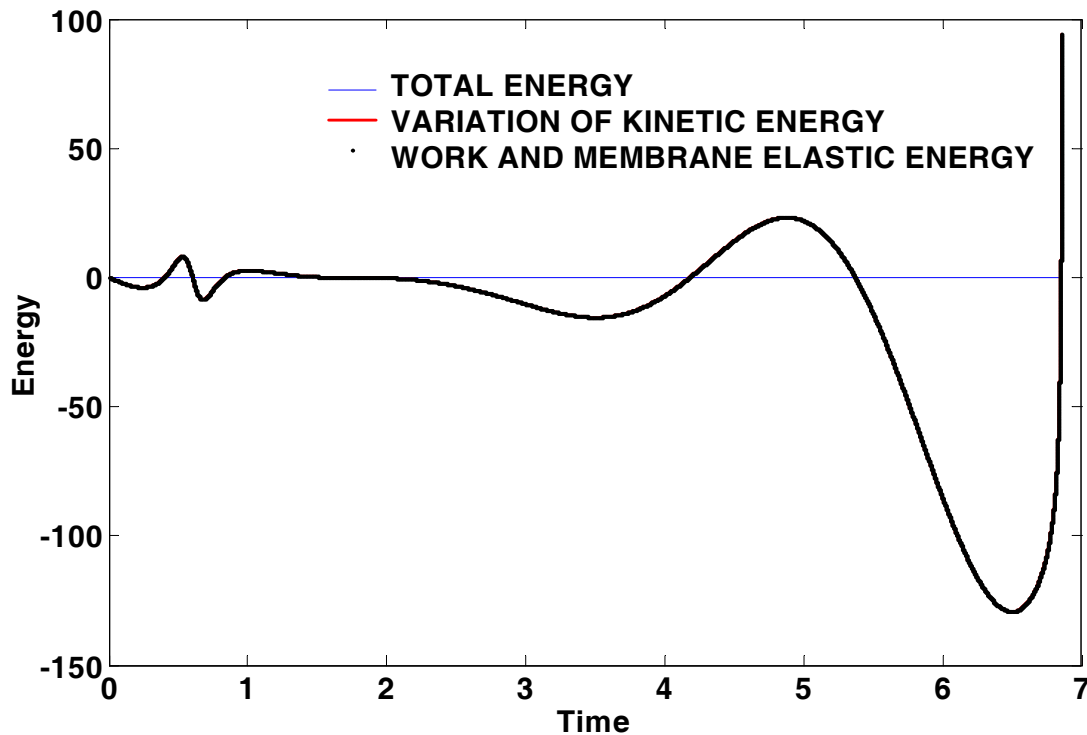
Σχήμα 3. Η συνολική ενέργεια της μικροφουσαλίδας συναρτήσει του χρόνου. Δεδομένα προσομοίωσης: R_{bal}=1.5 \mu m , G_s=18 MPa , \alpha=0.5 , \delta=15 nm , \rho_l=998 kg/m^3 , P_{st}=1 atm , v_f=2.4 MHz , \epsilon_{inf}=12 , \gamma=1.4 , αριθμός στοιχείων 100.
