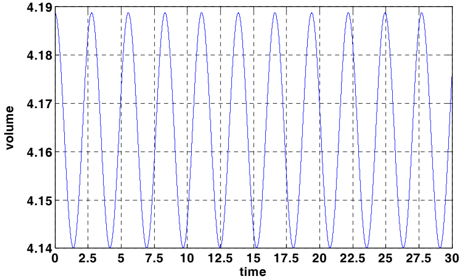
Σχήμα 2. Ο όγκος της μικροφουσαλίδας σε συνάρτηση του χρόνου για γραμμική διαταραχή. Δεδομένα προσομοίωσης: R_{bal}=1.5 \mu m , G_s=18 \text{ MPa} , \alpha=0.5 , \delta=15 \text{ nm} , \rho_l=998 \text{ kg/m}^3 , P_{st}=1 \text{ atm} , \nu_f=2.4 \text{ MHz} , \varepsilon_{inf}=0.05 , \gamma=1.4 , αριθμός στοιχείων 60.
