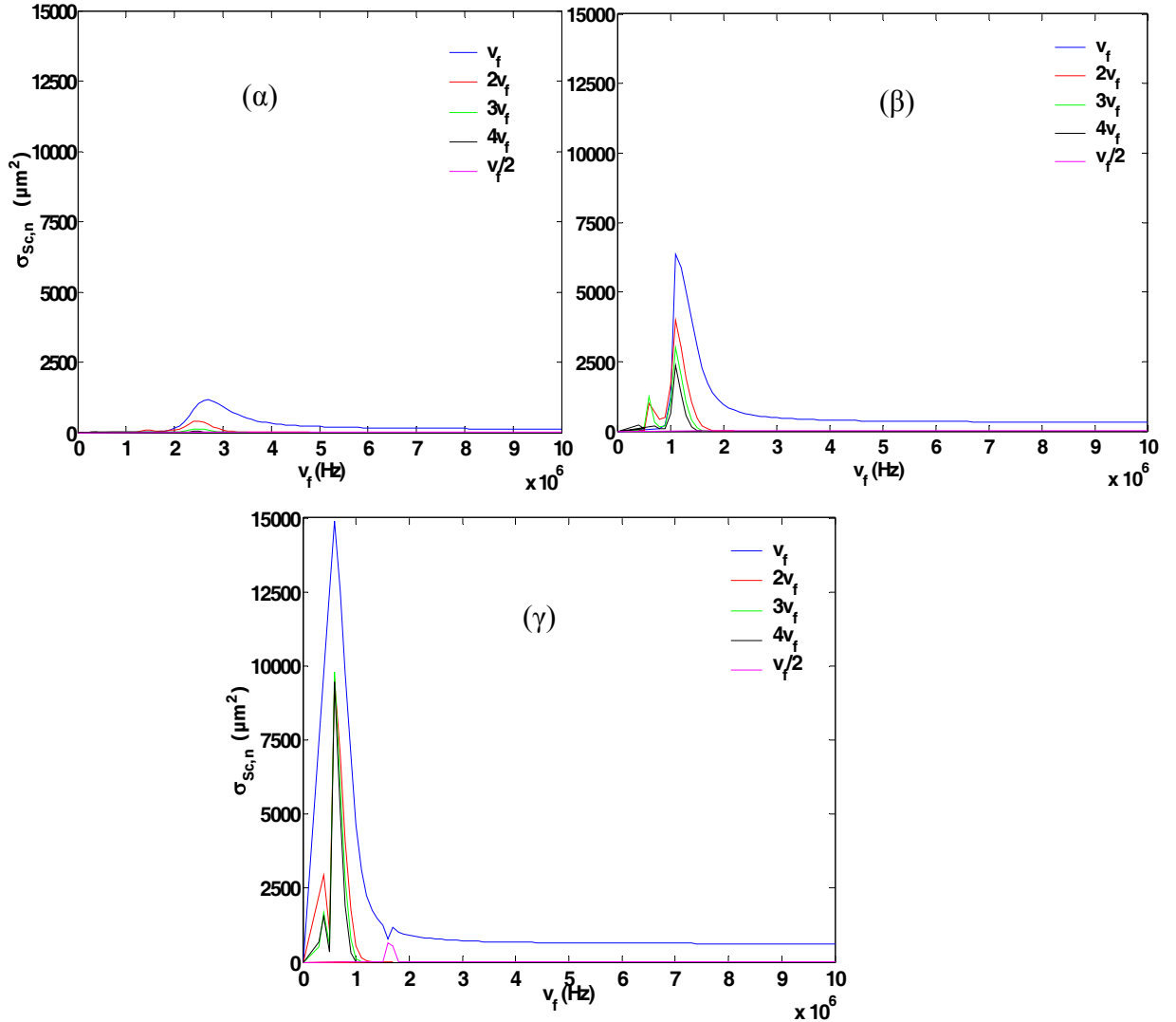
Σχήμα 7. Το \sigma_{Sc,n} σε συνάρτηση της εξωτερικής συχνότητας για α) \alpha=3 \cdot 10^{-6} m β) \alpha=5 \cdot 10^{-6} m, γ) \alpha=7 \cdot 10^{-6} m. Δεδομένα προσομοίωσης: \gamma=1.4 , P_{inf}=101325 Pa, \rho_l=998 kg/m 3 , s_1=0.04 kg/s 2 , s_2=0.005 kg/s 2 , \mu_l=0.001 kgm -1 s -1 , C_l=1500 m/s, G_s=35 MPa, \mu_s=0.6 kgm -1 s -1 , \delta=15 \cdot 10^{-9} m, E_{inf}=2.05 . u_r(t=0)|_{r=1} = u_r(t=0)|_{r=a_{bal}} = 0
