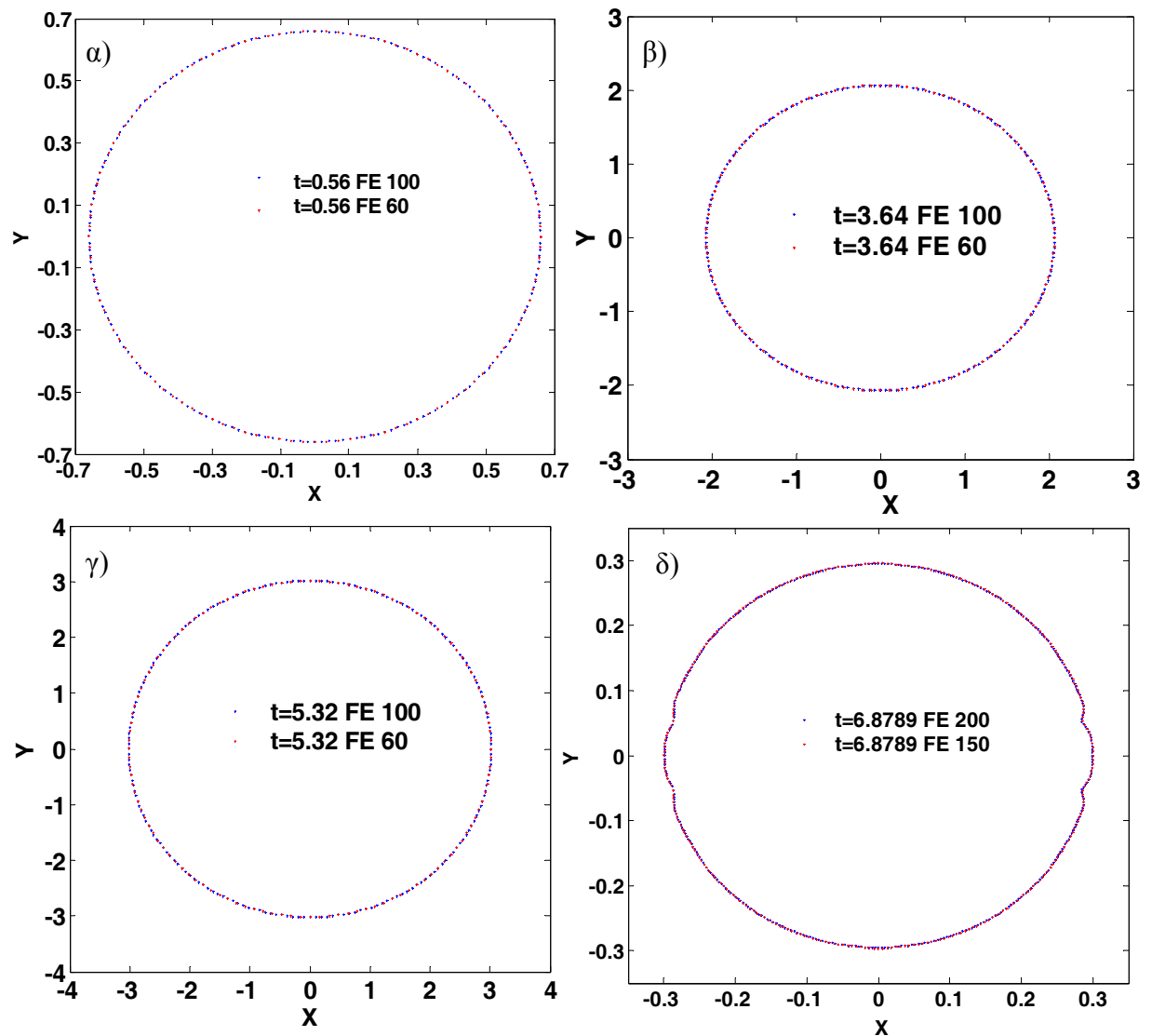
Σχήμα 4. Η ανεξαρτησία της λύσης με την πυκνωση του πλέγματος. Δεδομένα προσομοίωσης: R_{bal}=1.5 \mu m , G_s=18 \text{ MPa} , \alpha=0.5 , \delta=15 \text{ nm} , \rho_l=998 \text{ kg/m}^3 , P_{st}=1 \text{ atm} , v_f=2.4 \text{ MHz} , \epsilon_{inf}=12 , \gamma=1.4 .
