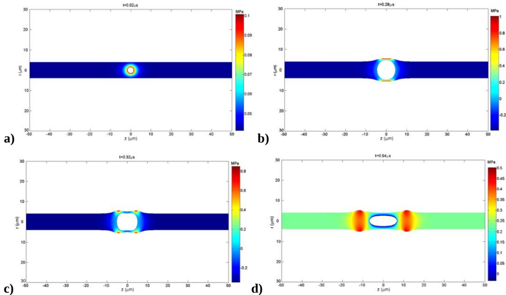
Εικόνα 1-5: Διαγράμματα κατανομής πίεσης εντός του αγγείου και της παραμόρφωσης της μικροφυσαλίδας CA: a) t=0.02 \mu s , b) t=0.28 \mu s μέγιστη διαστολή του αγγείου, c) t=0.32 \mu s μέγιστη διαστολή της μικροφυσαλίδας και d) t=0.54 \mu s .
